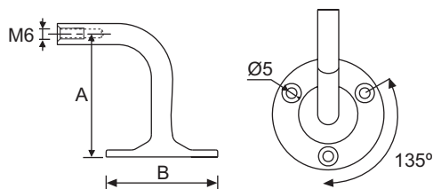
APOYO DE ATORNILLAR 90° SIMPLE
