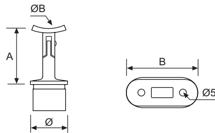
APOYO ÁNGULO VARIABLE
