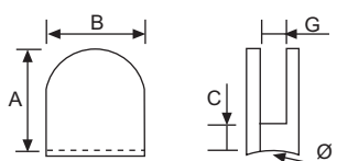
GRAPA CÓNCAVA
