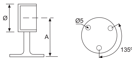
SOPORTE TERMINAL RECTO
