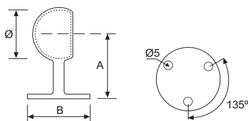
SOPORTE TERMINAL REDONDO
