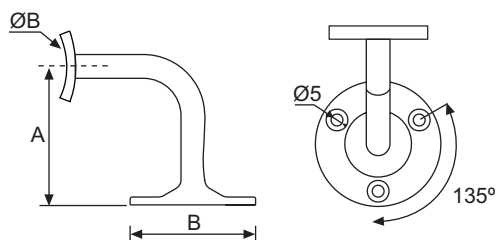
APOYO TUBO 90°
