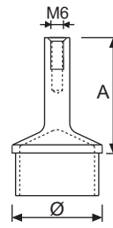
APOYO DE ATORNILLAR RECTO SIMPLE
